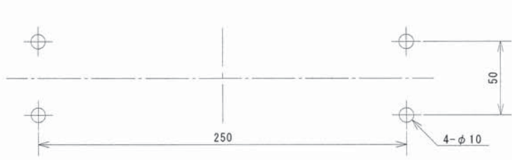
機器固定穴寸法
