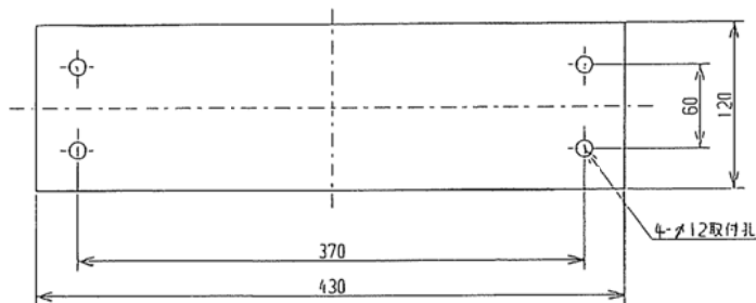
取付足寸法図
