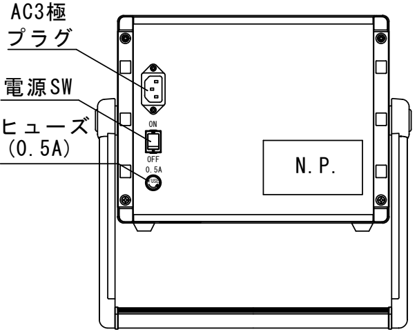
背面図
