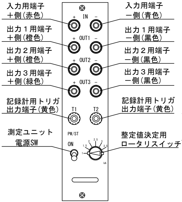
ソケット色およびユニット前面詳細図
