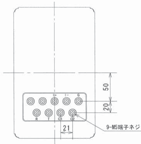
裏面端子図
