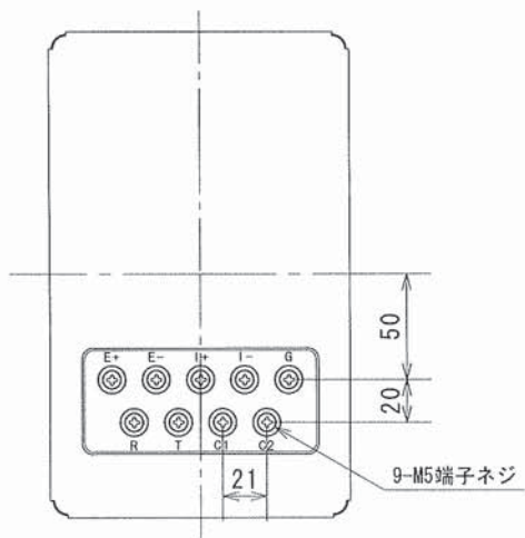
裏面端子図
