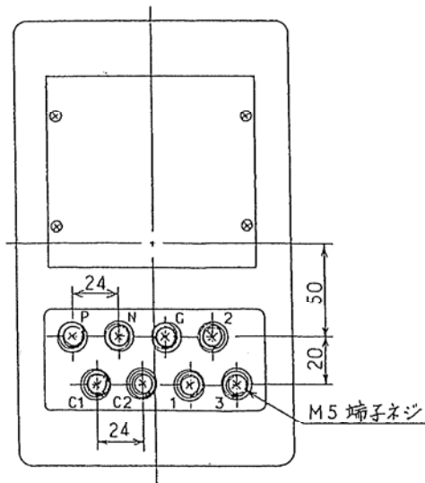
裏面端子図
