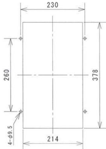
パネルカット (Scale 1/8)
