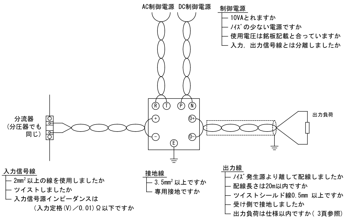
図 4 配線の確認
