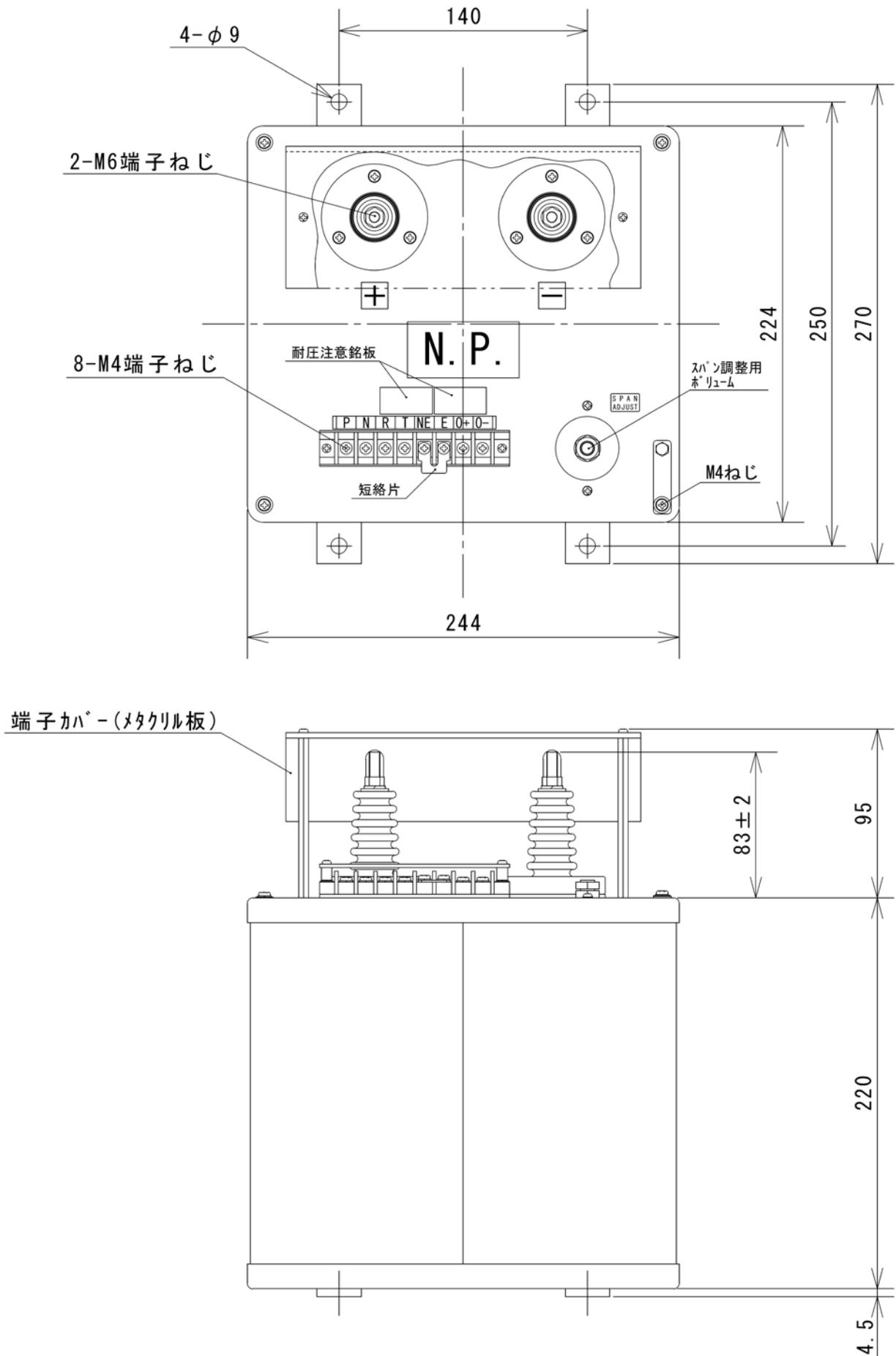
付図2 アイソレータ 外形寸法図
