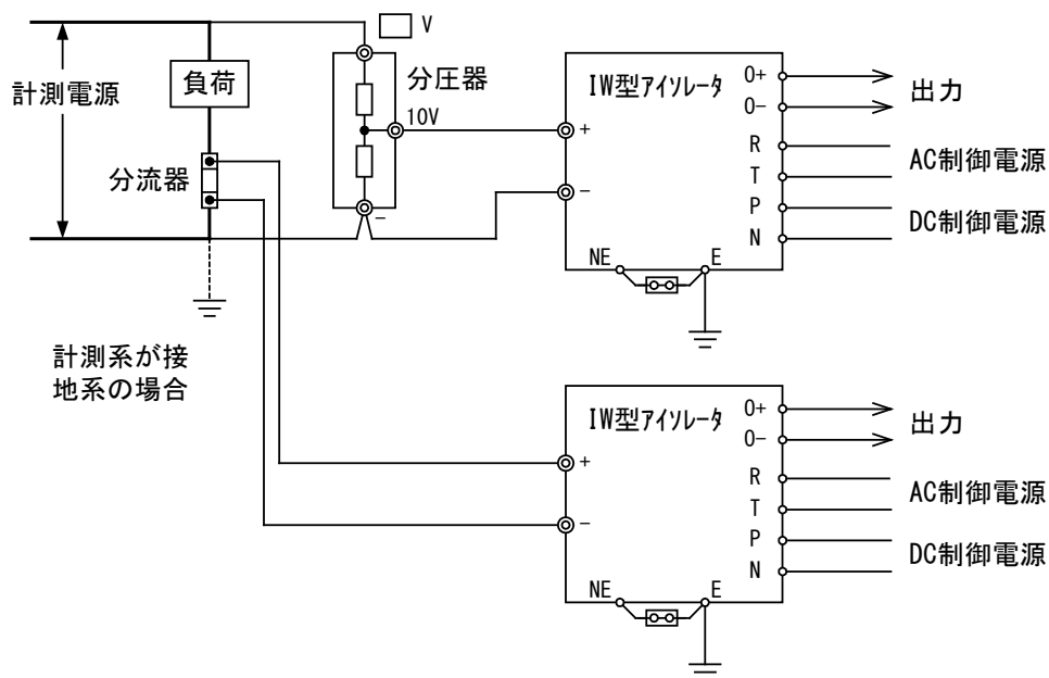
図 2 入力回路の接続
