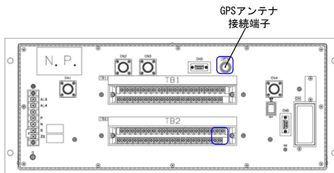
装置背面のGPSアンテナ接続端子
