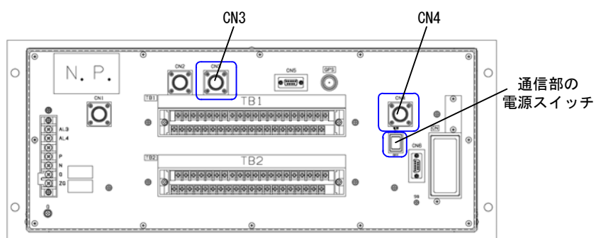
装置背面の CN3, CN4 および通信部の電源スイッチ
