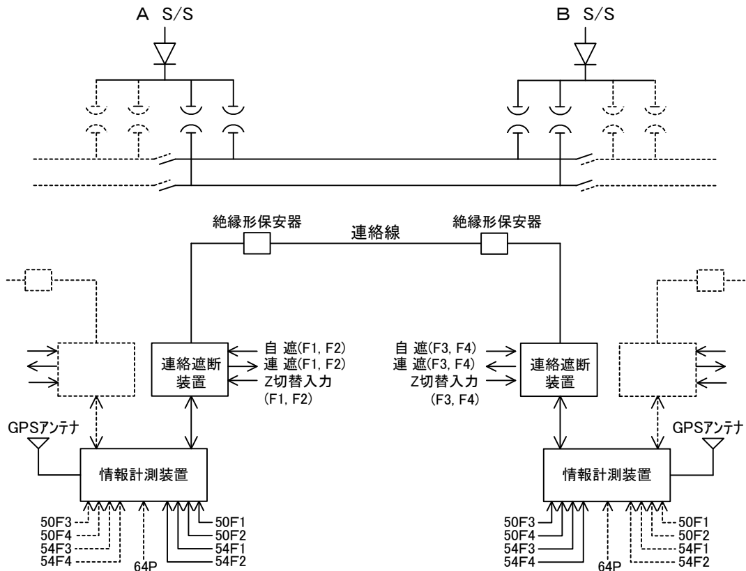
図6-2 システムブロック図
