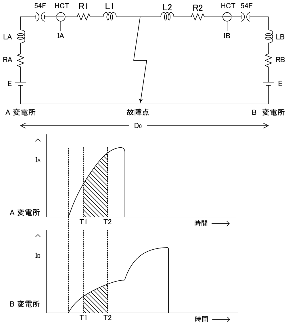
図 6 - 1 原理図
