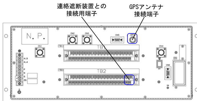
装置背面の GPS アンテナ接続端子および連絡遮断装置との接続用端子
