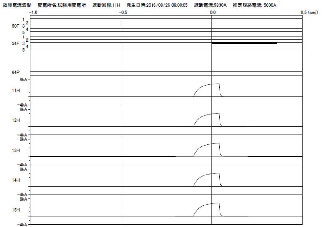
故障電流波形 (50F, 54F, 64P の動作表示) 印刷例
