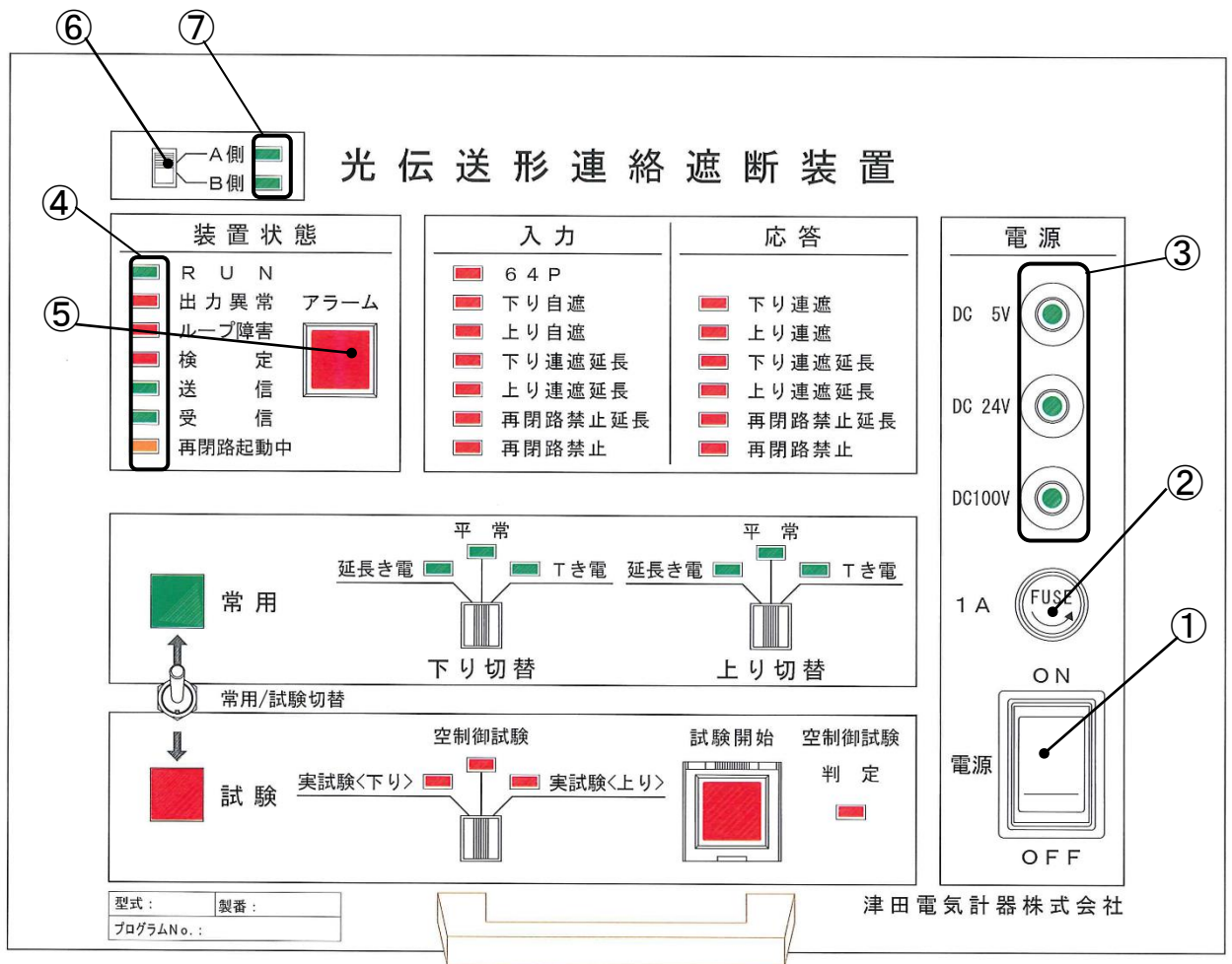
図 4-1 (b). 装置前面パネル(HRO-11H-1 型 再閉路禁止入出力機能 有りタイプ)
