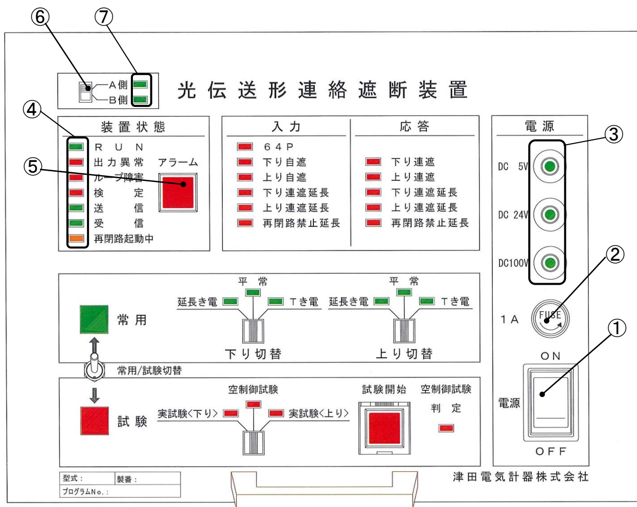
図 4-1(a). 装置前面パネル(HRO-11H-1 型 再閉路禁止入出力機能 無しタイプ)
