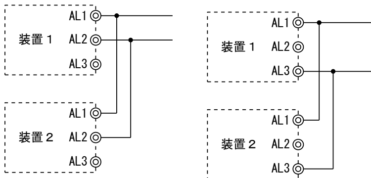
図 6-3. 装置異常出力接続方法 (2 台以上の装置使用時)
