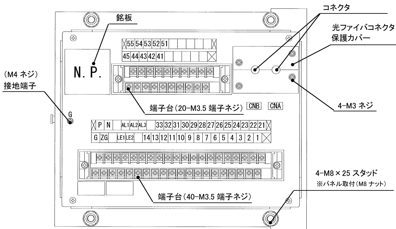
図 4-2. 装置背面図
