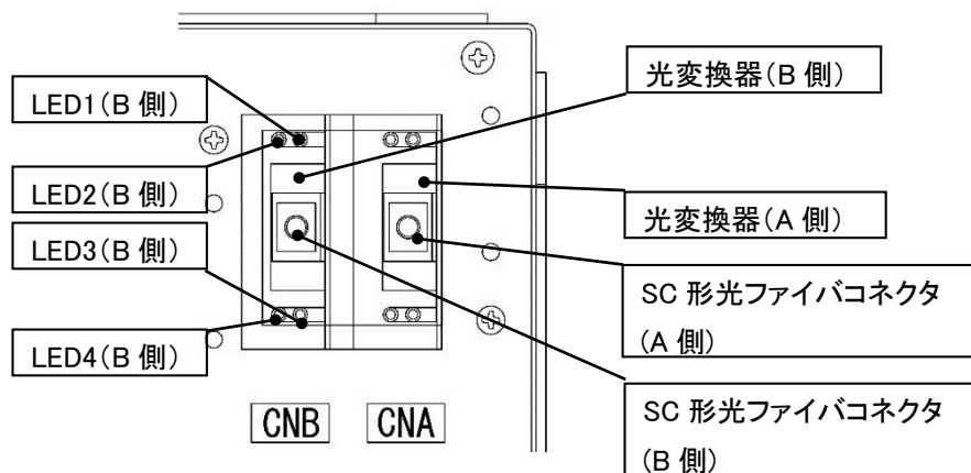
図 4-3. 光ファイバコネクタ保護カバー取り外し時
