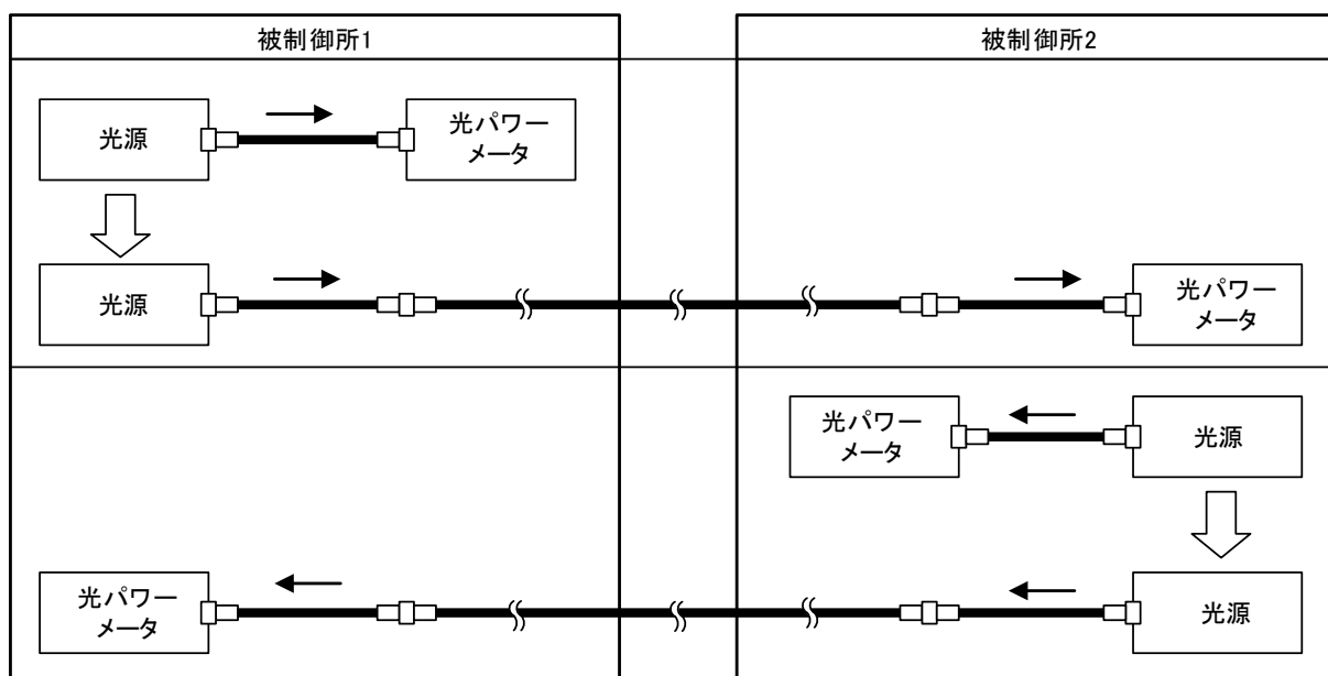
図 5-1. 連絡線の減衰特性の確認
