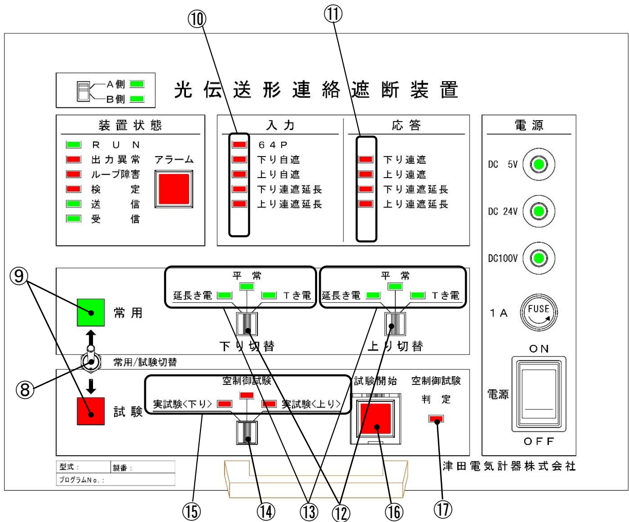
図 4-1 (d). 装置前面パネル(HRO-12H-1 型 再閉路禁止入出力機能 無しタイプ)
