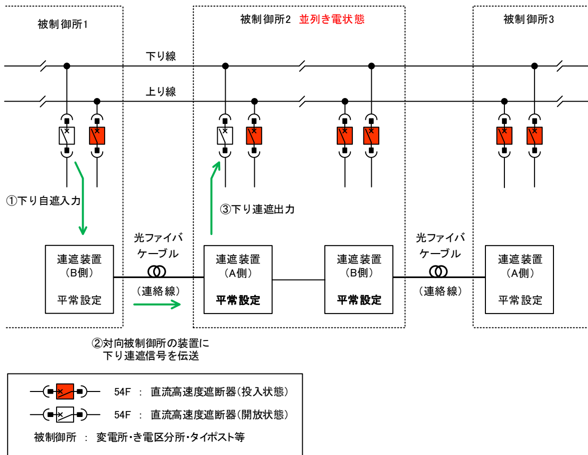
図 1-3. 並列き電時の連遮装置の動作例(「平常」設定時)
