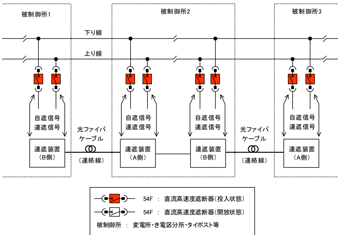
図 1-2. 光伝送形連絡遮断装置の構成例
