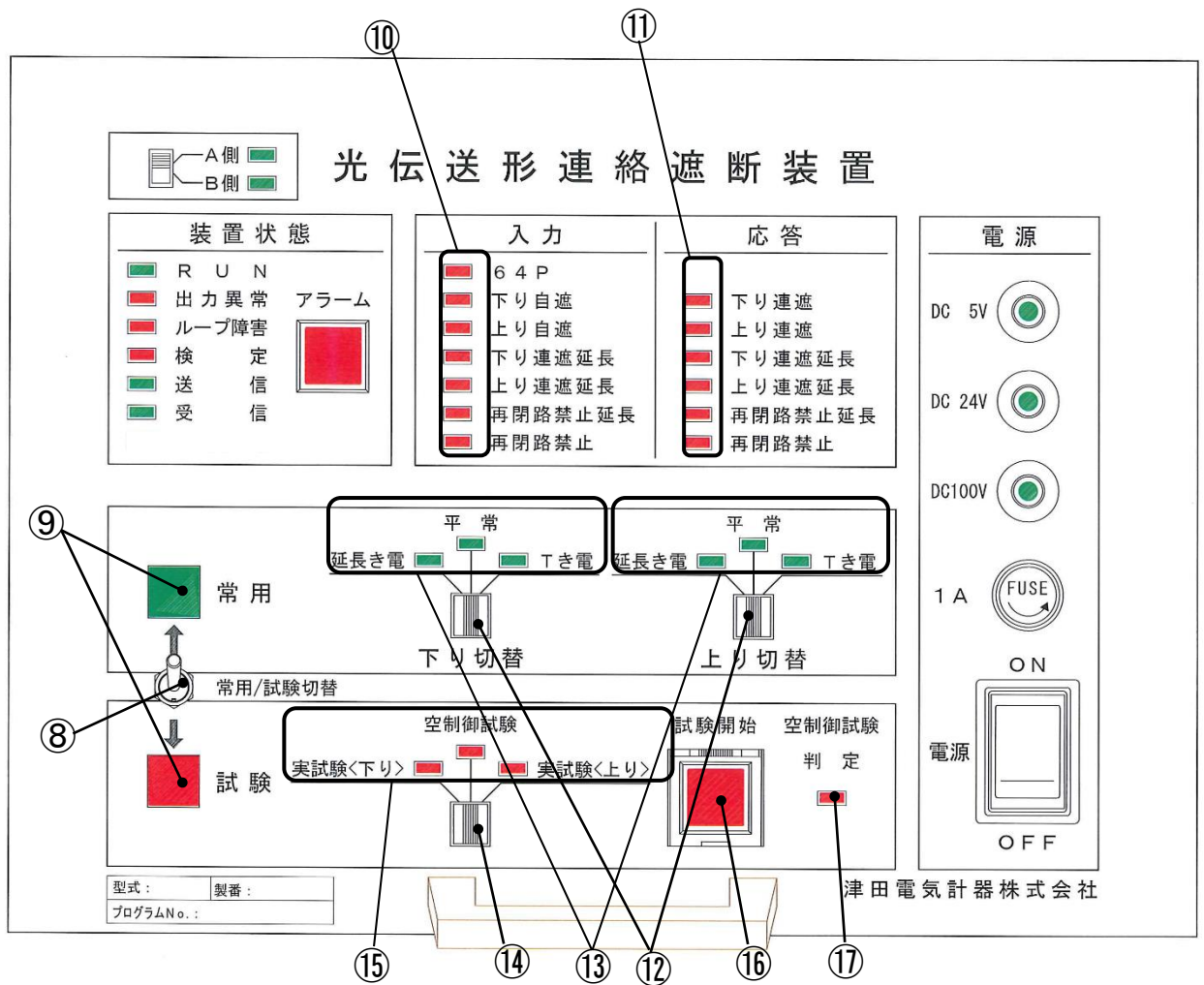
図 4-1 (c). 装置前面パネル(HRO-12H-1 型 再閉路禁止入出力機能 有りタイプ)
