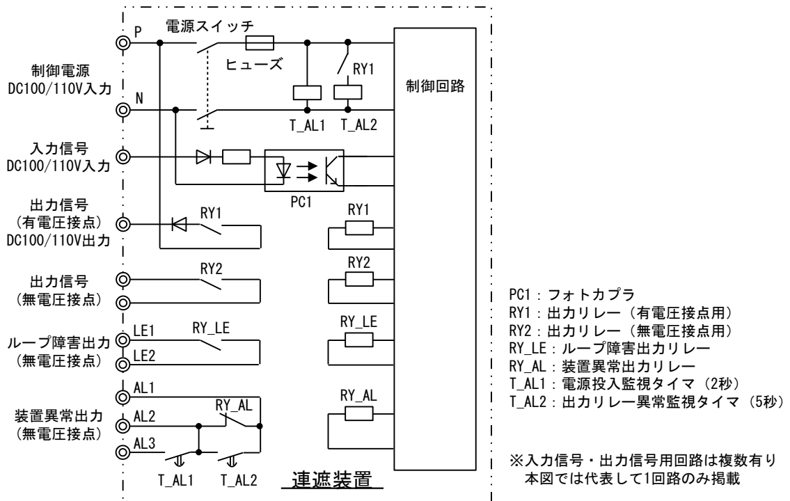
図 6-1. 入出力信号回路
