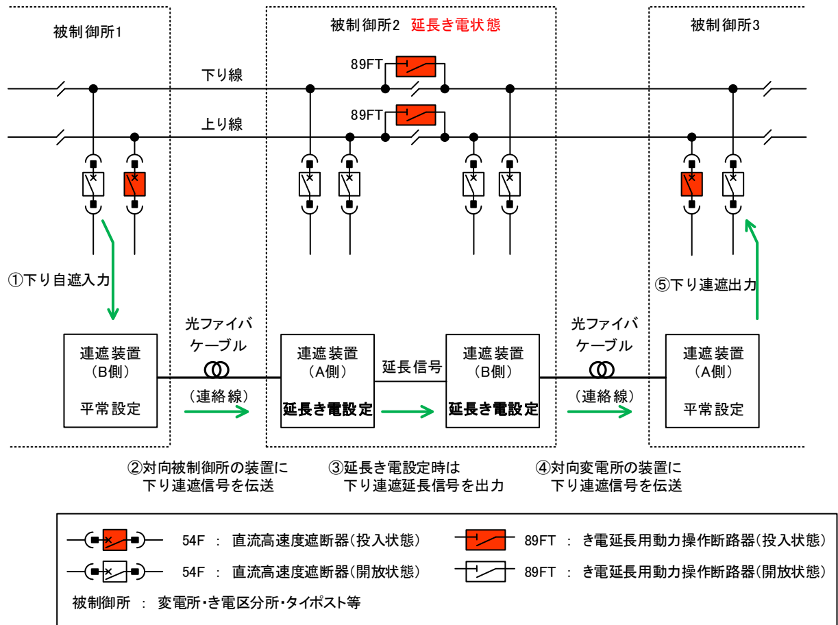
図 1-4. 延長き電時の連遮装置の動作例(延長き電設定時)
