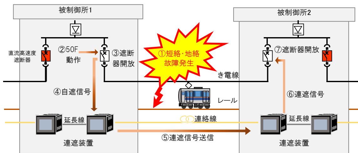
図 1-1. 連遮装置の目的
