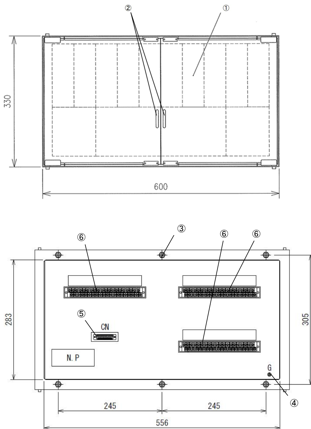
図 2. 故障選択装置
