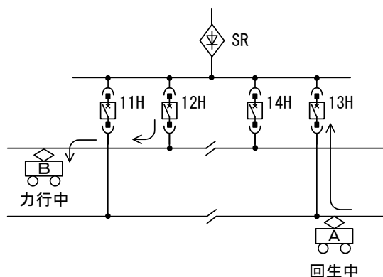
図 32. 回生電流
