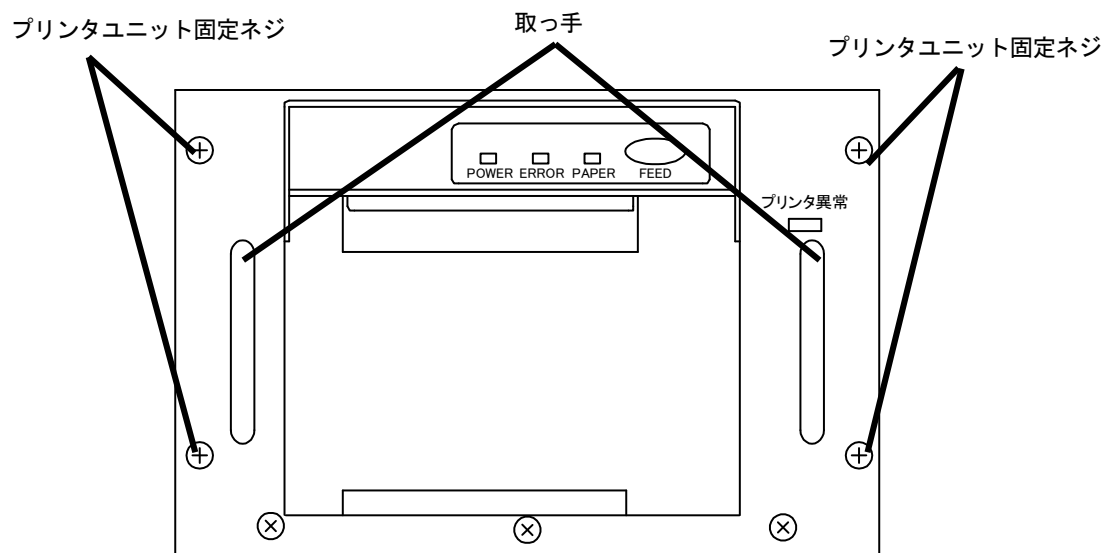
図 29. プリンタユニット取り外し方法
