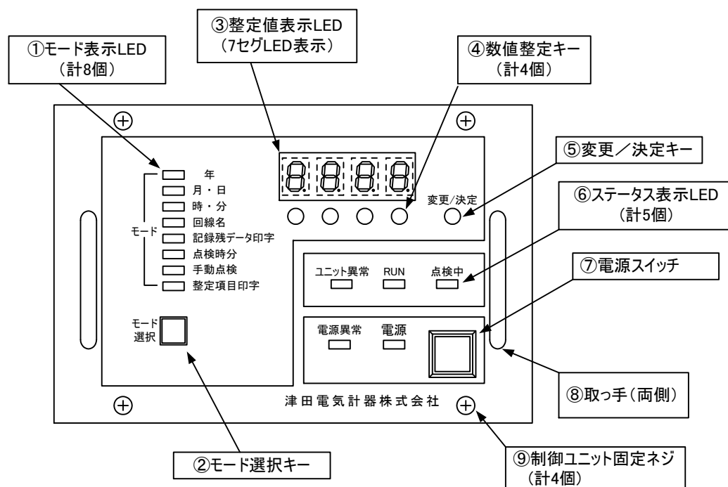
図 5. 制御ユニット 前面パネル
