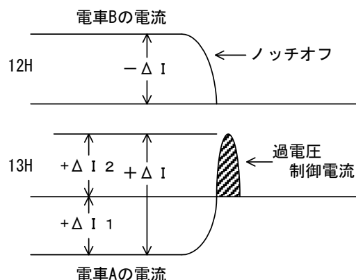
図 33. 回生 OFF 時の電流変化
