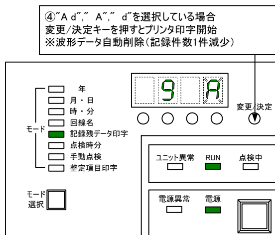
図17. “記録残データ”の操作方法
