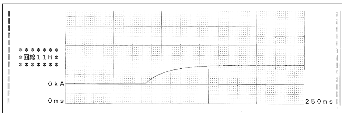
図 20. 事故電流波形アナログデータ
