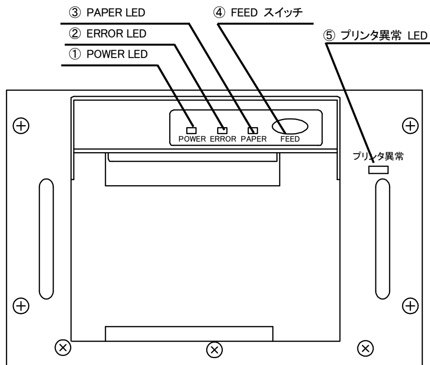
図 6. プリントユニット 前面パネル
