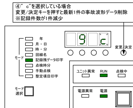
図17. “記録残データ”の操作方法
