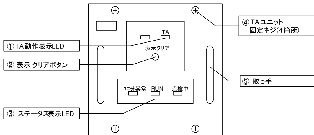
図 30. TA ユニット前面パネル
