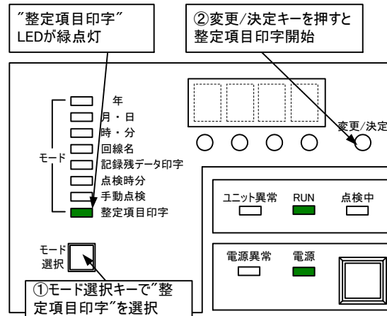
図 22. “整定項目印字”の操作方法
