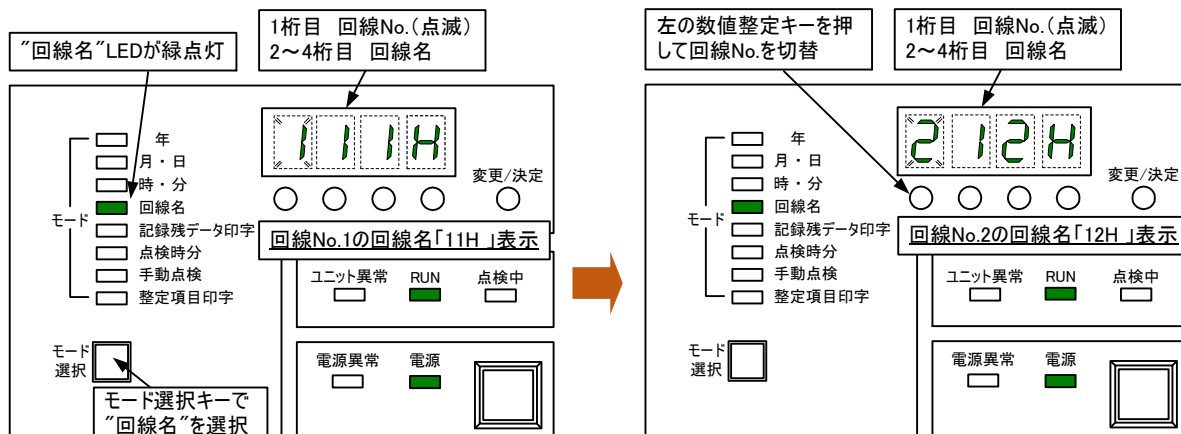
図 25. “回線名”の表示
