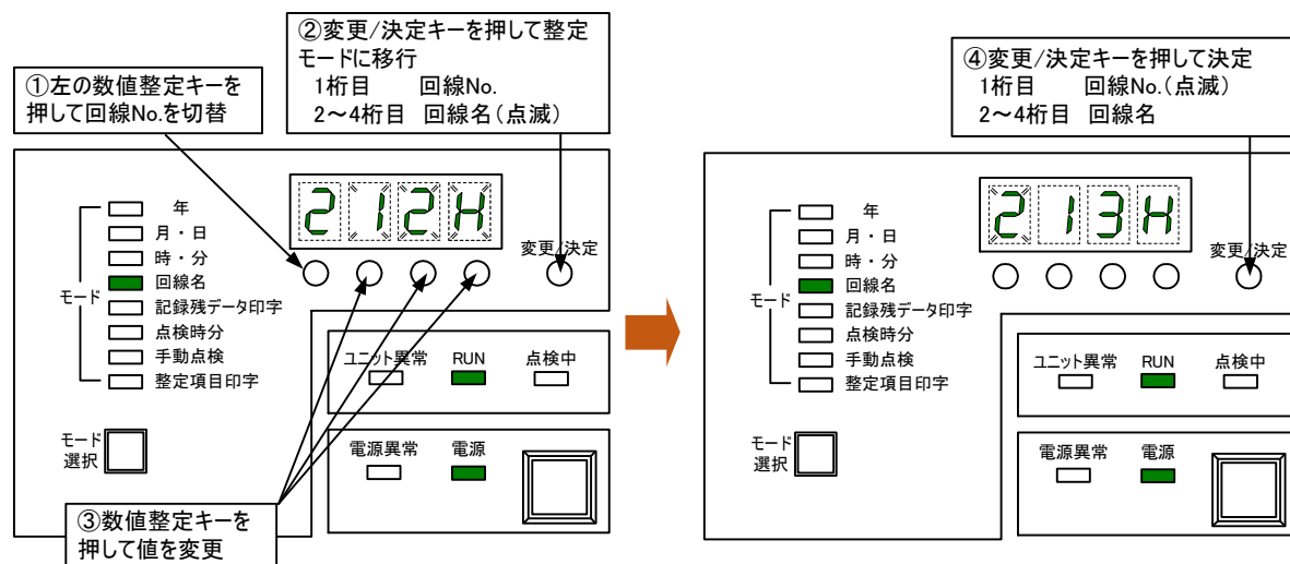
図 26. “回線名”の整定
