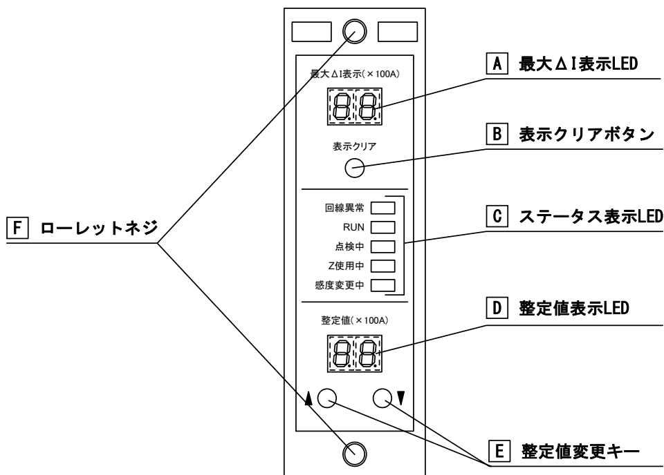
図 16. \Delta I ユニット 前面パネル
