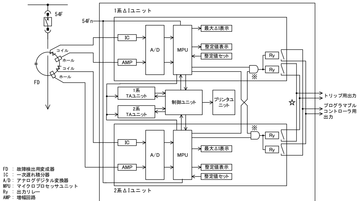
図1. ブロック図
