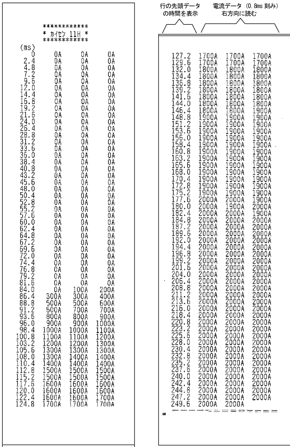
図 21. 事故電流波形デジタルデータ
