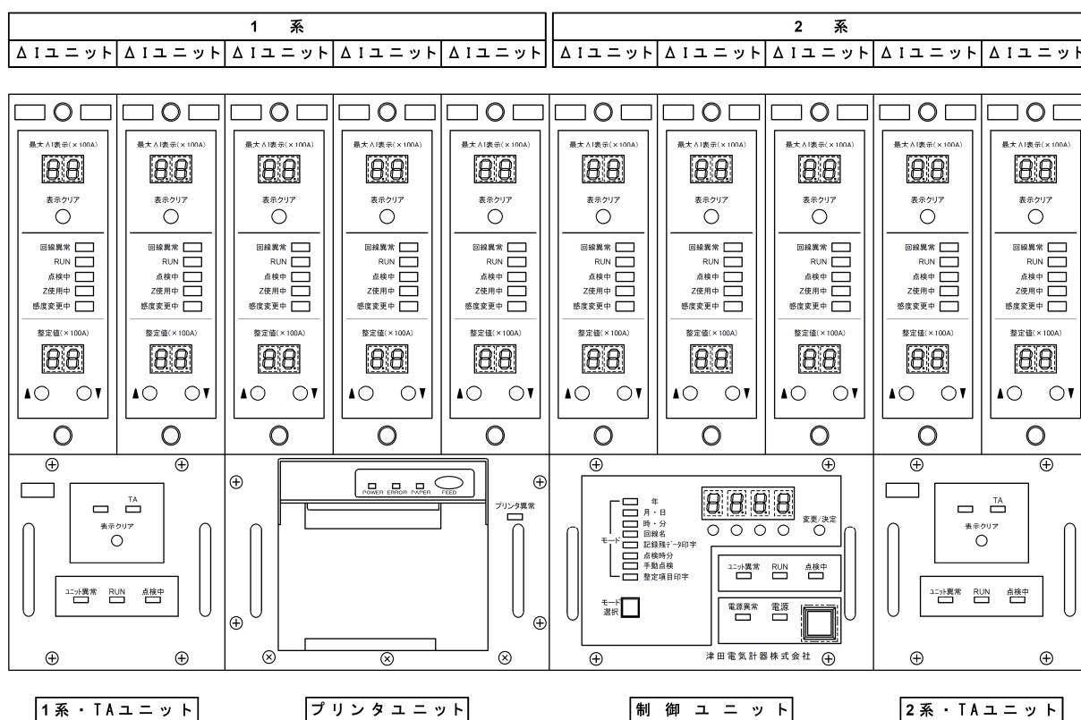
図 3. 故障選択装置のユニット構成例（全ユニット実装時）
