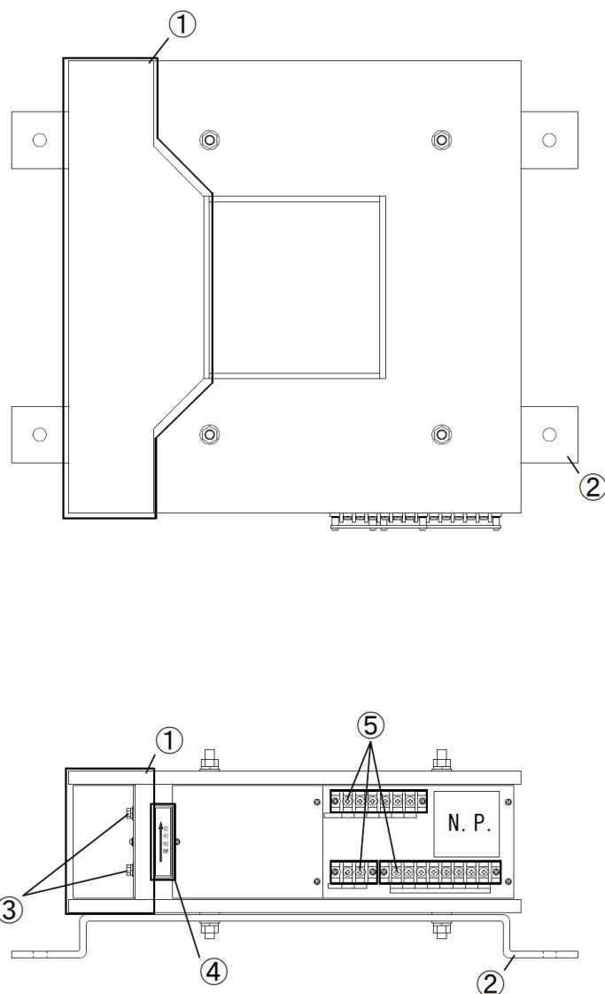
図 10. 故障検出用変成器 (DF-10 型)
