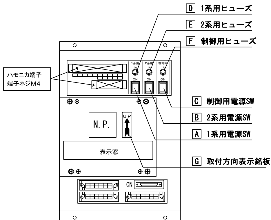
図 8. 電源部 (SF-3T2 型) の操作面
