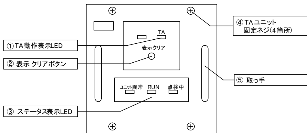
図 7. TA ユニット前面パネル
