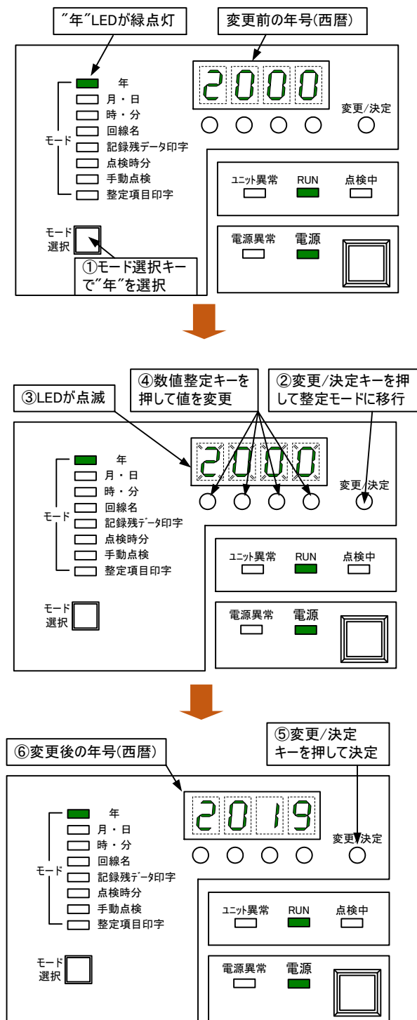
図 24. “年”の整定方法
