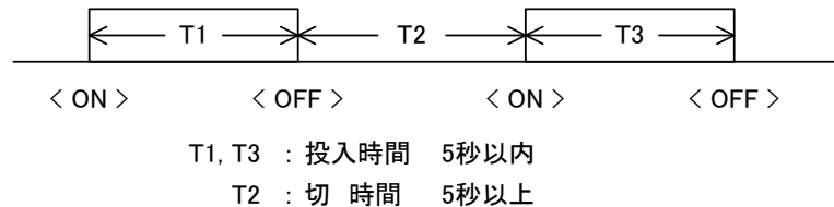
図 37. 試験器操作時のスイッチ入切サイクル
