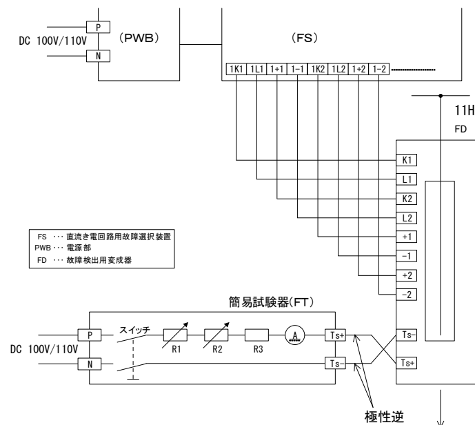
図 38. 回生失効時の不動作確認試験回路
