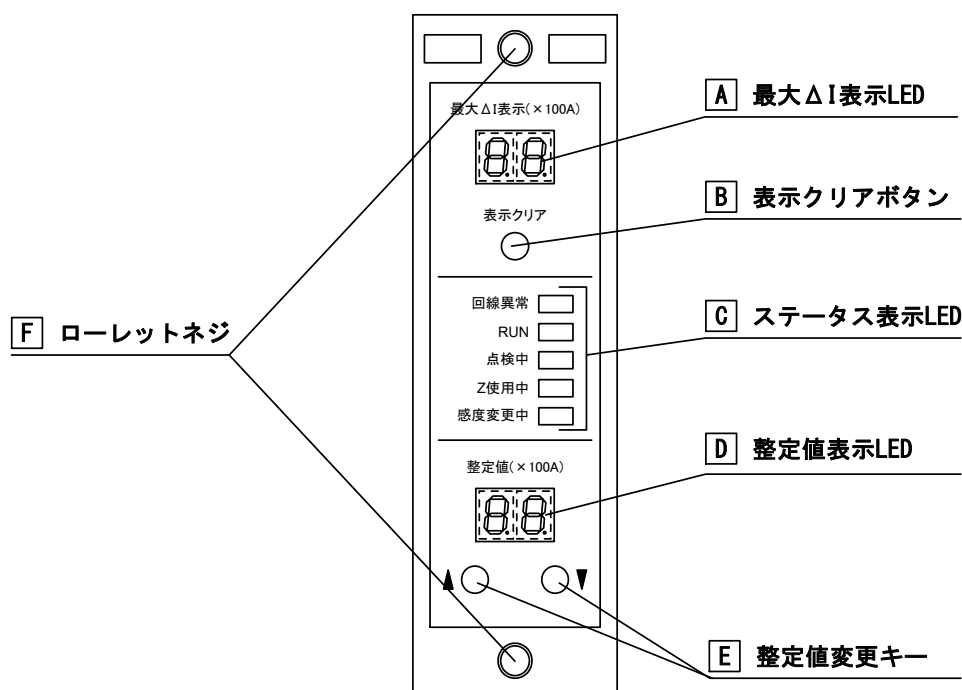
図 4. \Delta I ユニット 前面パネル
