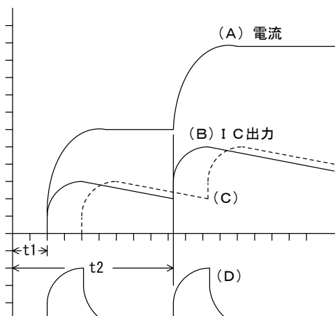
図 31. \Delta I 分離機能
