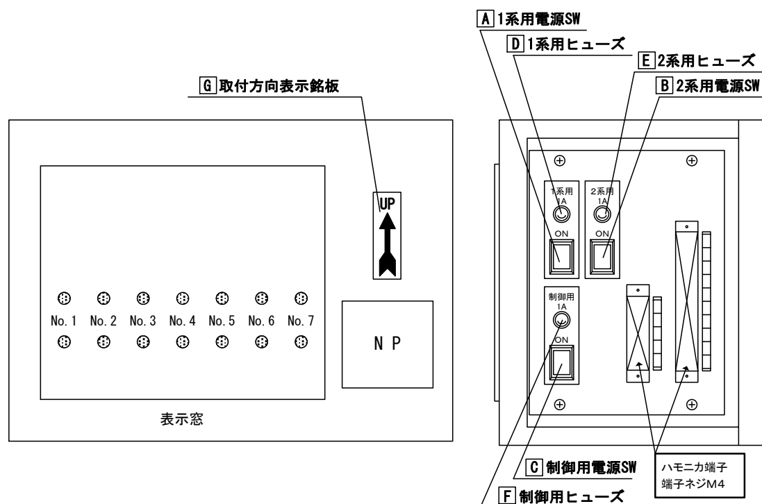
図 9. 電源部 (SF-3Y2 型/SF-32 型) の操作面
