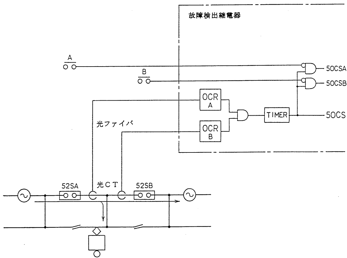
図1 原理図
